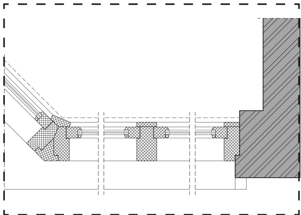
Horizontaal referentiedetail G1 - woninggevel verdieping oorspronkelijke toestand houten kozijn met schuiframen
