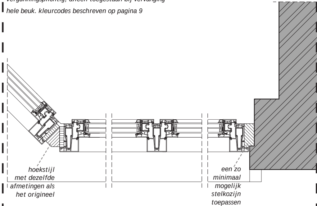
Horizontaal referentiedetail G6 - woninggevel verdieping vervanging door kunststof kozijnen en ramen met isole- rende beglazing
