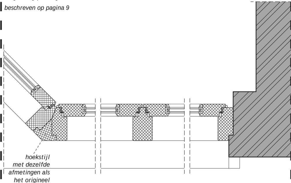
Horizontaal referentiedetail G4/5 - woninggevel verdieping vervanging door houten kozijnen met nieuwe houten ramen voor- zien van dubbelglas en optioneel verholen ventilatie
