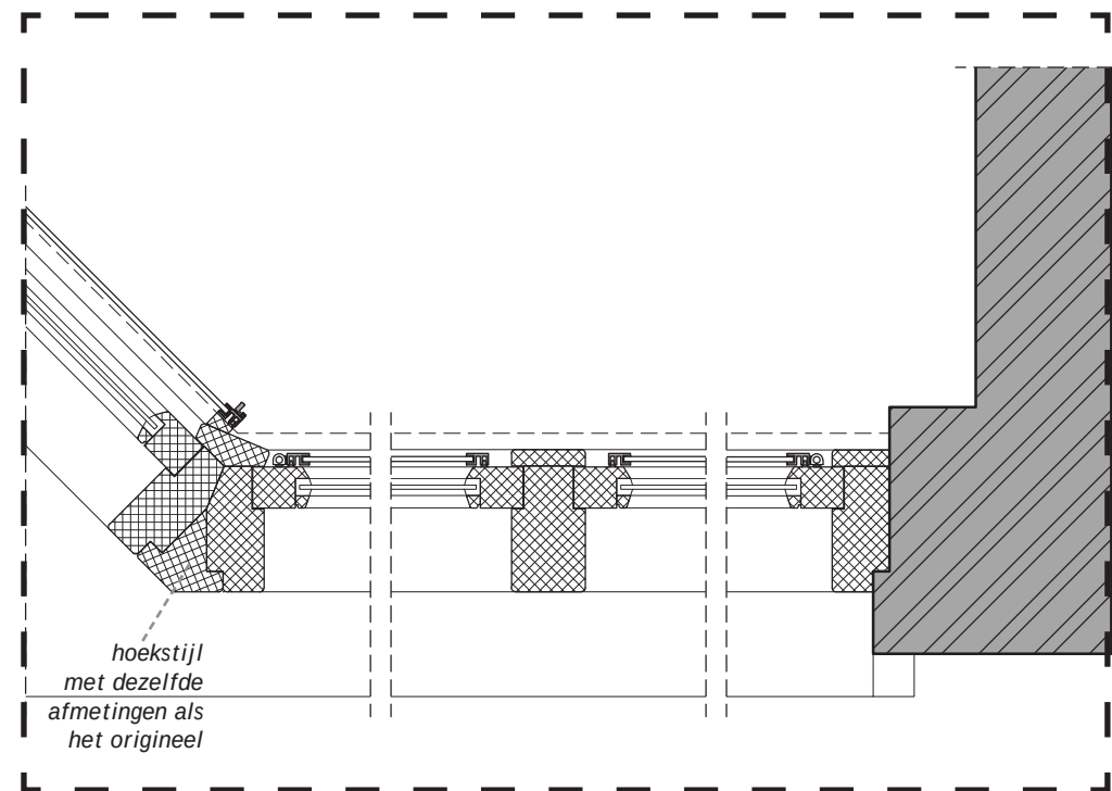
Horizontaal referentiedetail G2 - woninggevel verdieping onderhoudsvariant: originele houten kozijnen met nieuwe achter- zetramen
