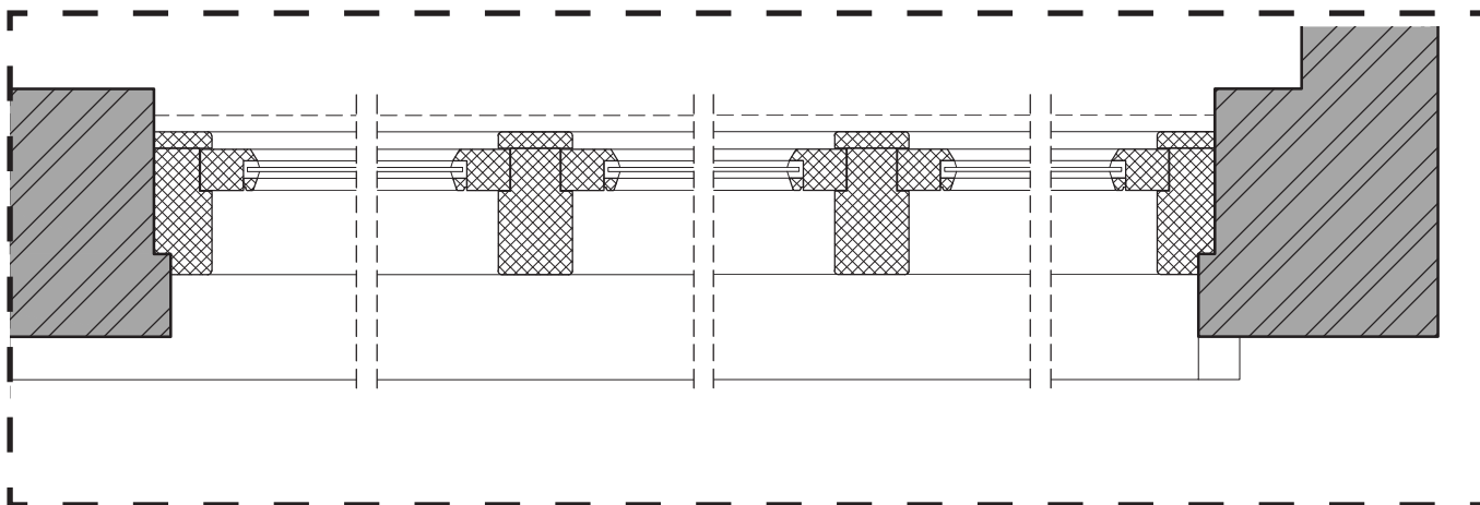
Referentiedetail E1 - woninggevel
