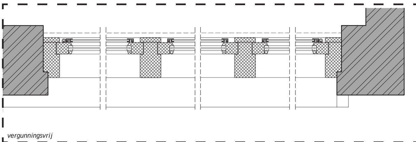
Referentiedetail E2/3 - woninggevel begane grond
