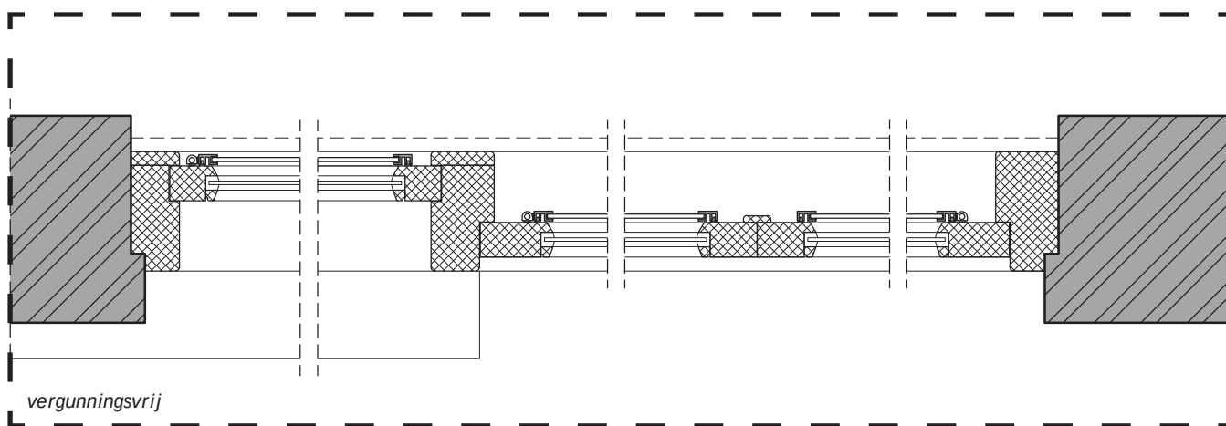
Horizontaal referentiedetail H2 - woninggevel dakverdieping onderhoudsvariant: originele houten kozijnen met nieuwe achter- zetramen
