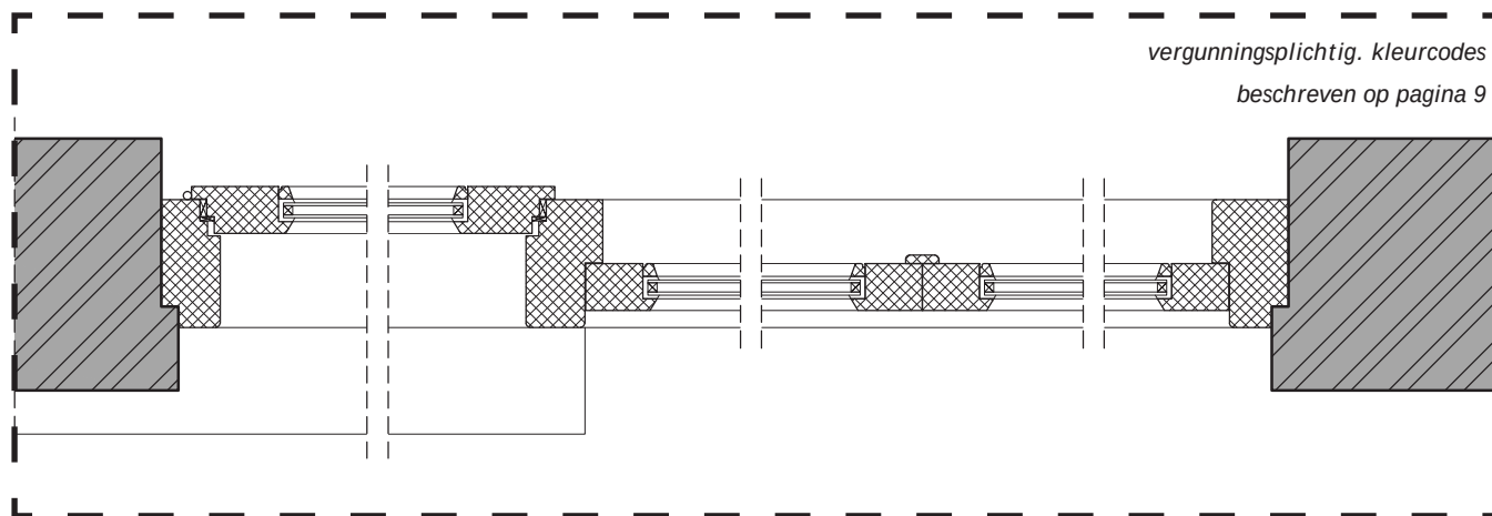
Horizontaal referentiedetail H4/5 - woninggevel dakverdieping vervanging door houten kozijnen met nieuwe houten ramen voorzien van dubbelglas en optioneel verholen ventilatie
