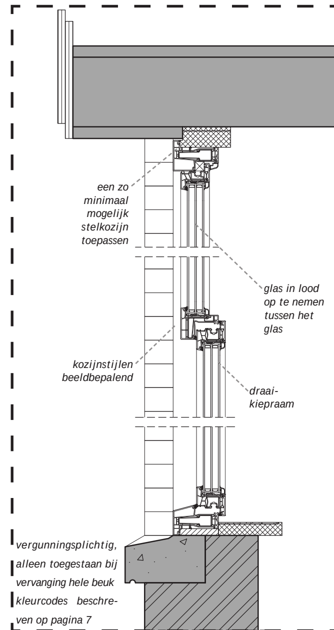
Referentiedetail C6 - woninggevel dakverdieping vervanging door kunststof kozijnen en ramen met isolerende beglazing
