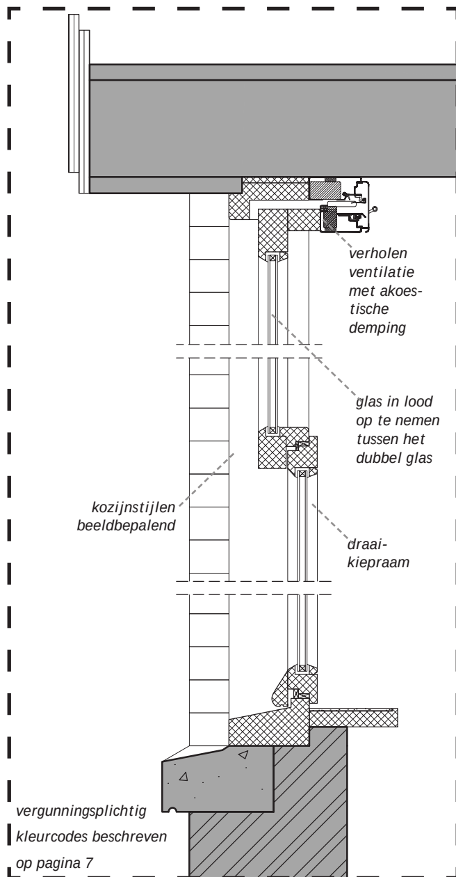
Referentiedetail C5 - woninggevel dakverdieping vervanging door houten kozijnen en nieuwe houten ramen met dubbel glas en met verholen ventilatie
