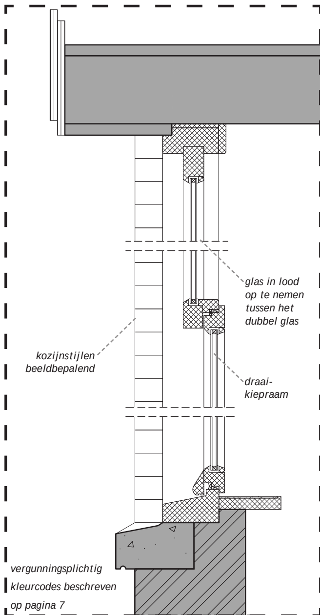
Referentiedetail C4 - woninggevel dakverdieping vervanging door houten kozijnen met nieuwe houten ramen voorzien van dubbelglas
