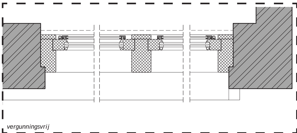
Referentiedetail E2/3 - woninggevel begane grond
